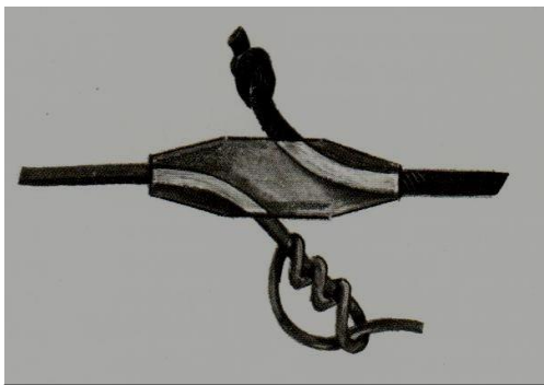
Collegamento del finale alla coda tramite "cast-connector"
