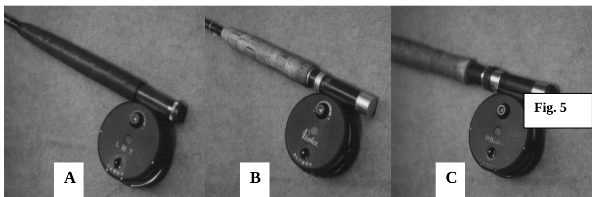
Fig. 5: particolare del bloccaggio con diversi portamulinelli. Risulta evidente come il tipo A (con vite inferiore a scomparsa) si presenti più compatto e porti il mulinello più vicino all'impugnatura. Per contro il tipo C (ad avvitamento superiore) posiziona il mulinello troppo lontano dall'impugnatura risultando particolarmente scomodo. Nel tipo B (ad anello) il pregio maggiore è sicuramente la leggerezza.
